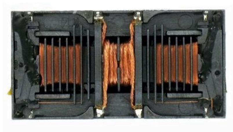
TMS91195CT TRASFORMATORE INVERTER PER LCD
